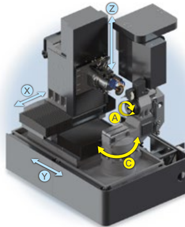
軸構成 Axis structure
