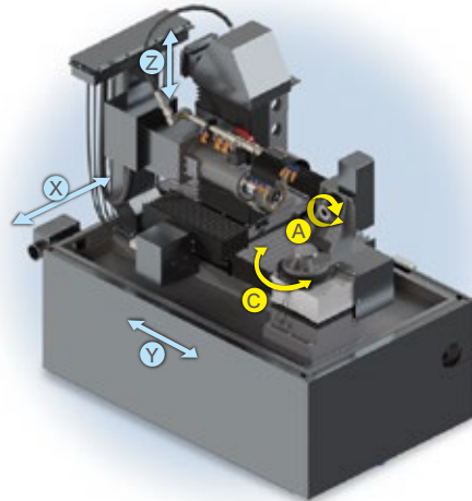
軸構成 Axis structure
