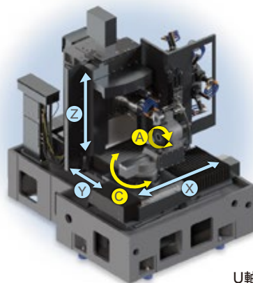
軸構成 Axis structure
